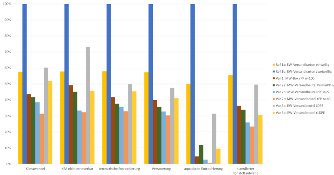
Abb. 3: Ergebnisse der verschiedenen Versandverpackungen (Ausgewählte Indikatoren)
